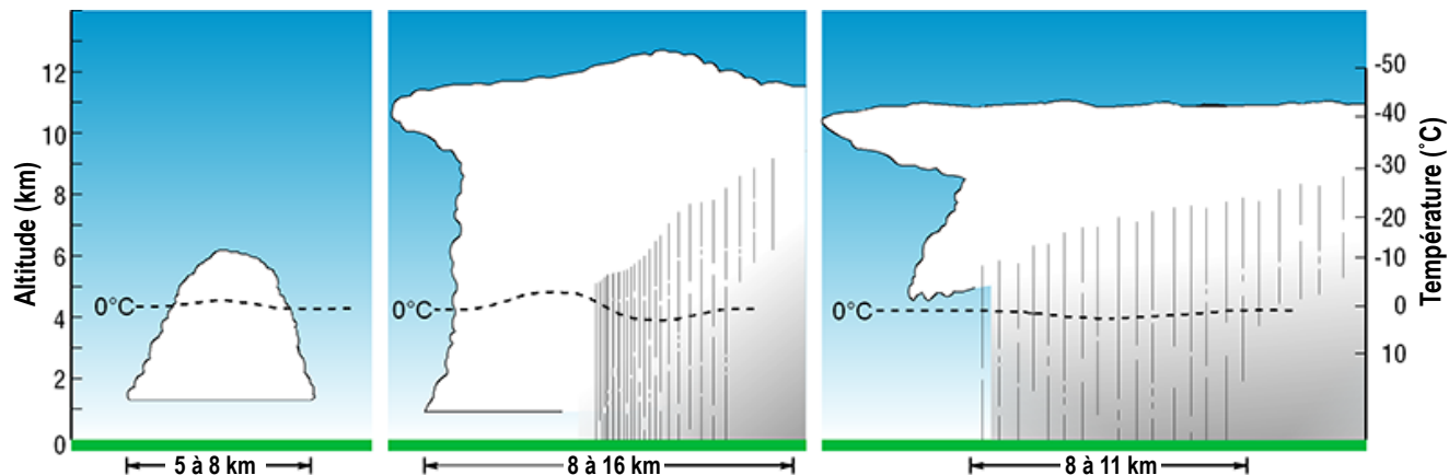
Trois stades d'un orage (avec l'aimable autorisation de la NOAA).
