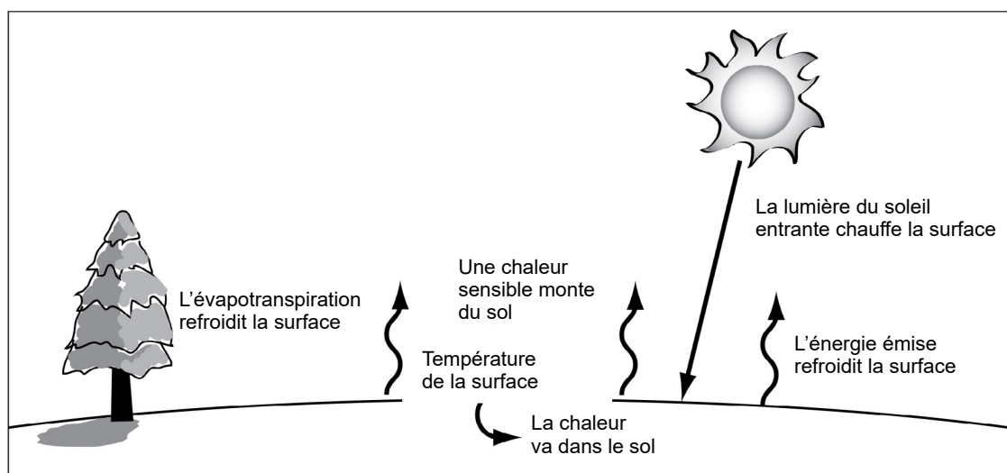
Répartition de l'énergie solaire par rapport à la température de surface de la Terre. Source : Lecture du protocole de GLOBE sur la température de surface (avec l'aimable autorisation de GLOBE).
