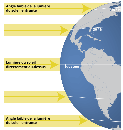
Lumière solaire entrante à diverses latitudes (Crédit : SA Geography)
